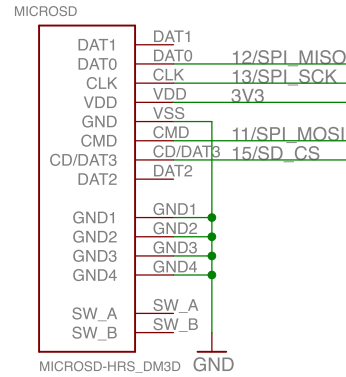
MICROSD-HRS_DM3D
