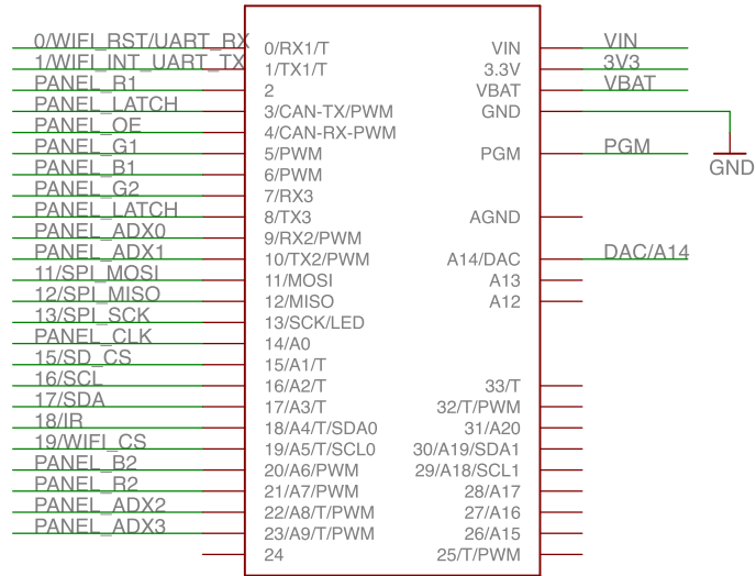
TEENSY_3.0_ALL-UUSB-A10-A11-AREF
